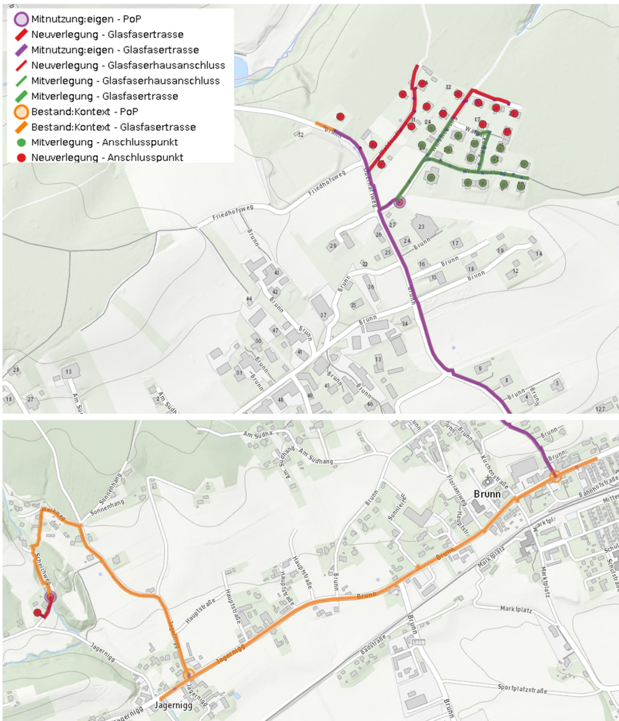
(Plandarstellung)
